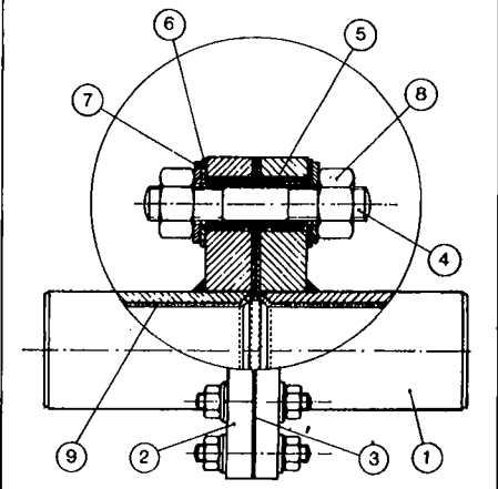
FIG. 23 - Giunto isolante a flangia
