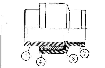
FIG. 22 - Giunto isolante per tubi gas
