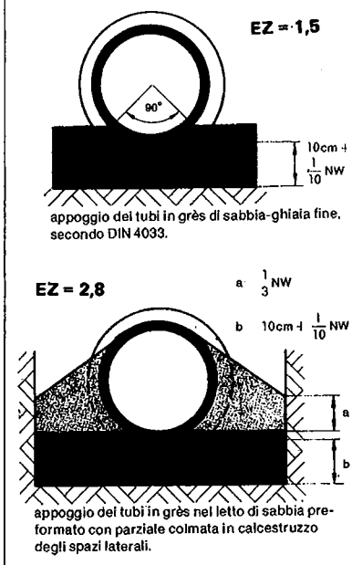
FIG. 30 - Tubazioni di grès. Posa su sabbia - Indici EZ
